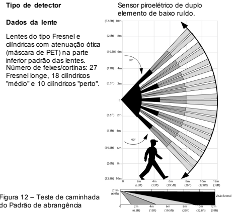
Figura 12 – Teste de caminhada do Padrão de abrangência
